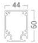
Querträger
